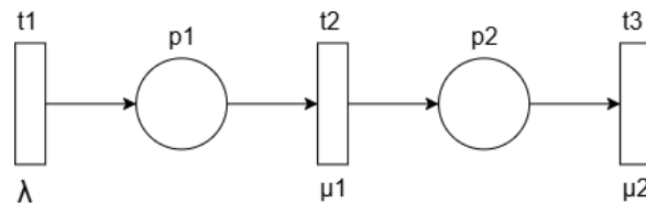
Figura 3.2: Modelul serie al rețelei Petri
