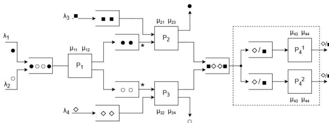
Figura 3.1: Reprezentarea schematică a sistemului de servire studiat
