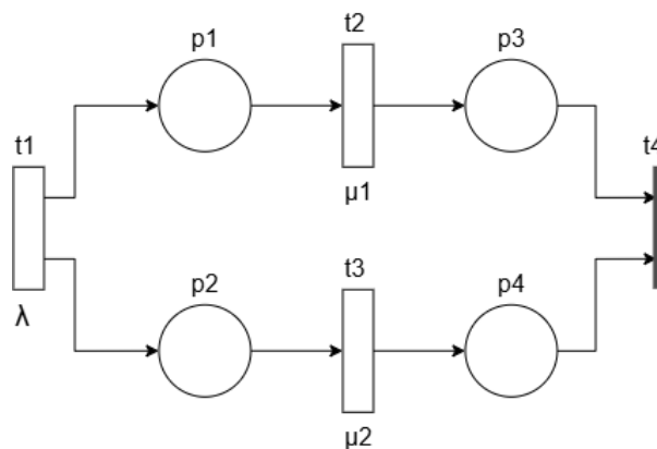
Figura 3.3: Modelul paralel al rețelei Petri
