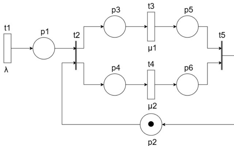
Figura 3.4: Modelul sincron al rețelei Petri
